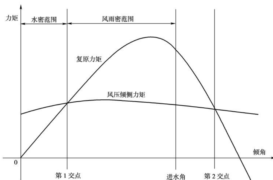
图 3.3.1.1 复原力矩和风压倾侧力矩曲线
