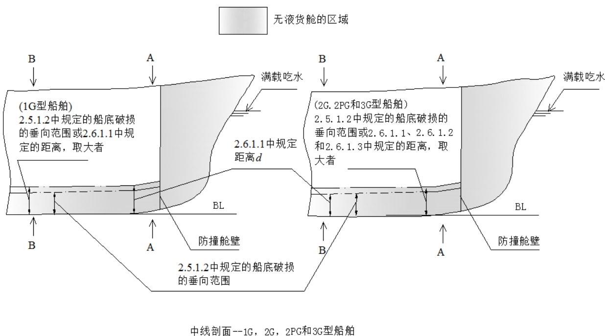
图 2.1 液货舱位置要求
