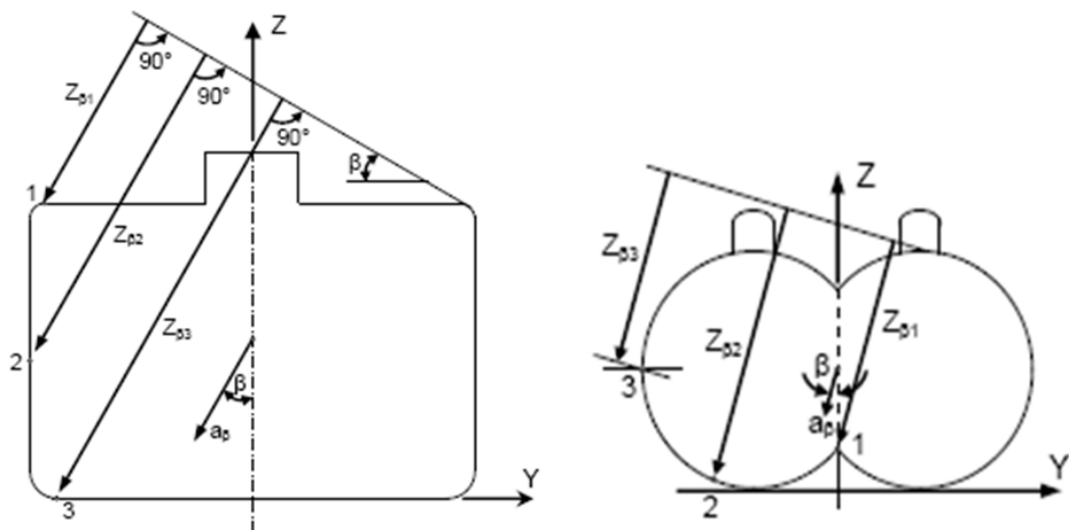
图4.22.3 (3) 点1、2和3的液体高度 Z_\beta 的确定
