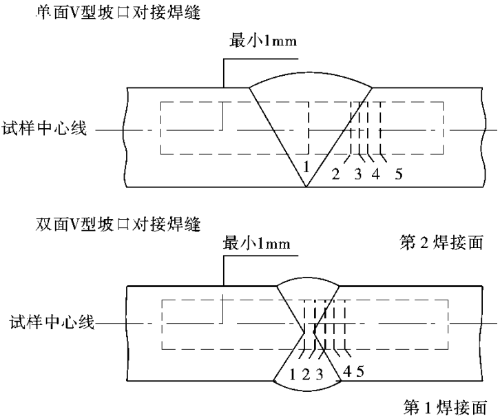
图 6.2 焊接试样的方向性
