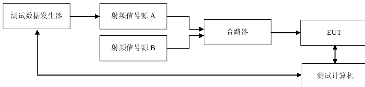
图7 多路信号源测试框图
