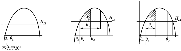
图 2 破损稳性
