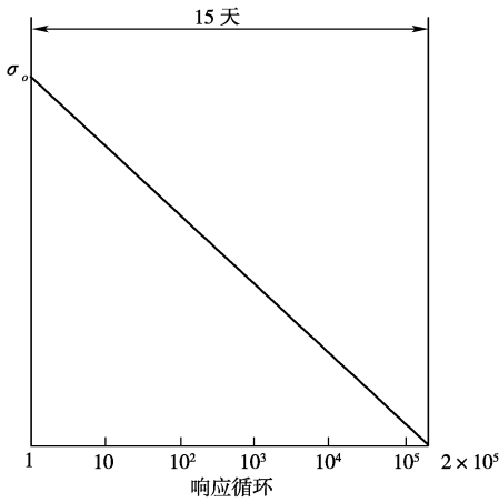
图 4.3 简化的载荷分布
