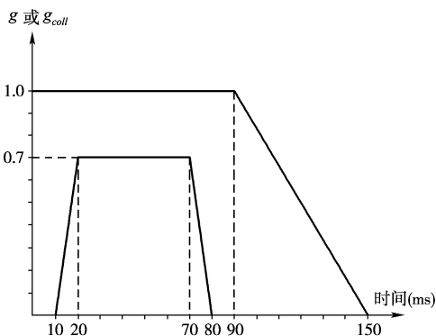
图 3.3 加速度与时间关系的包络线
