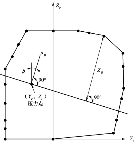
图 4.2 内部压头确定
