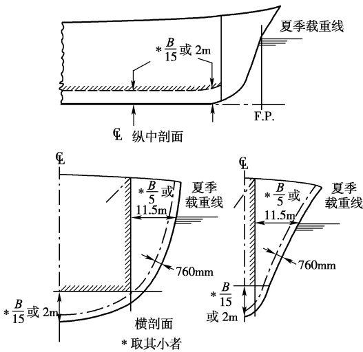
图 2.1 液舱位置要求 (按 2.6 规定)
