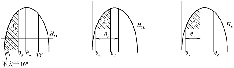
图 1 完整稳性
