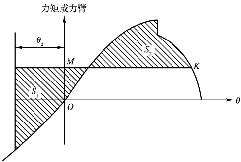
图 1 静稳性曲线
