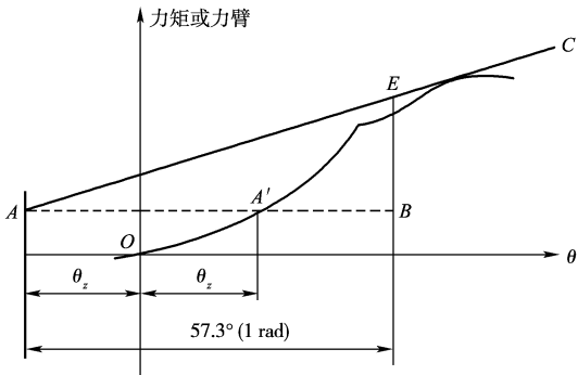
图 2 动稳性曲线
