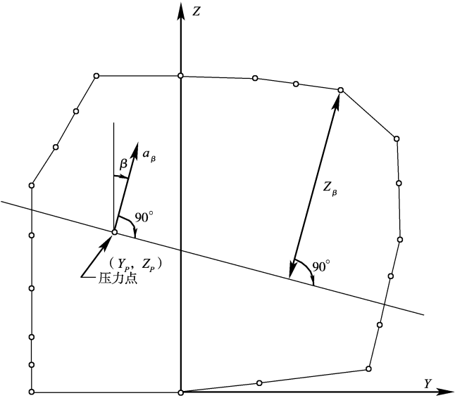
图 6.4.2 内部压头的确定
