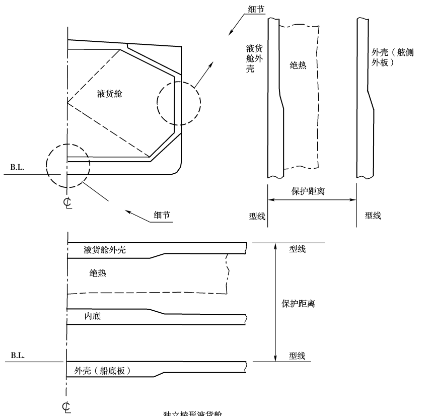
独立棱形液货舱
