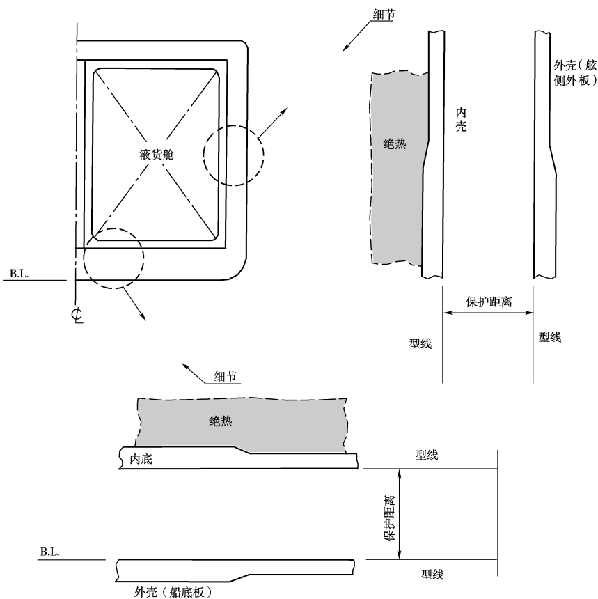
半薄膜液货舱
