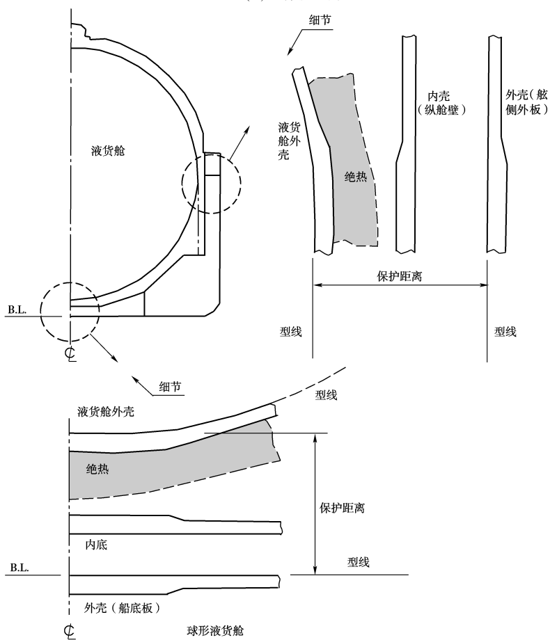
图 2.5(d) 保护距离
