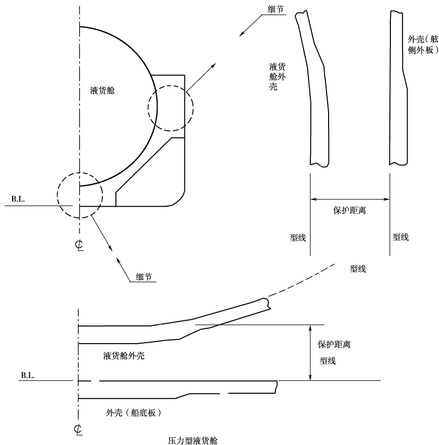
图 2.5(e) 保护距离
