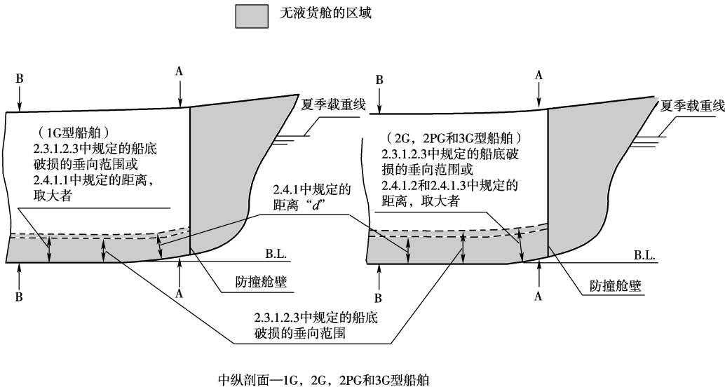
图 2.1 液货舱位置要求
