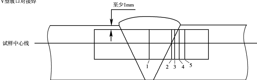
V型坡口对接焊
