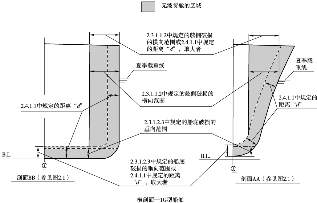
图 2.2 液货舱位置要求
