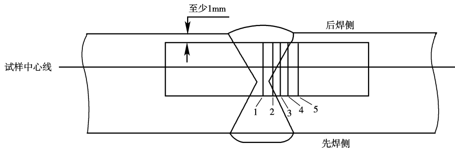
图 16.2 焊接试样的方向性
