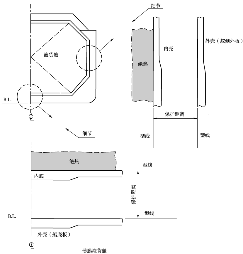
图 2.5(c) 保护距离
