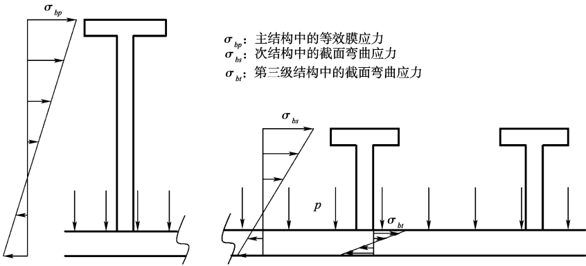
图 1 3 种截面应力的定义 (应力 \sigma_{bp} 和 \sigma_{bs} 垂直于所示的横截面)
