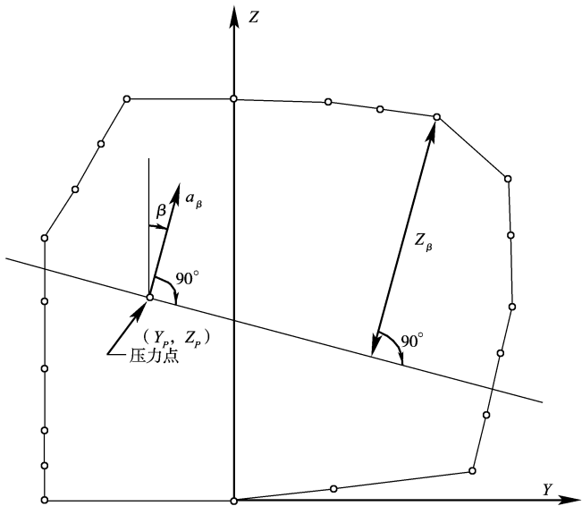
图 4.2 内部压头的确定
