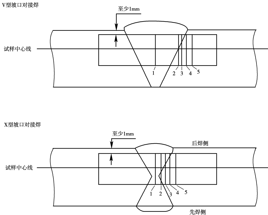
图 6.2 焊接试样的方向性
