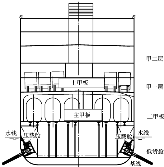
图 5(1) 车辆装载的典型布置
