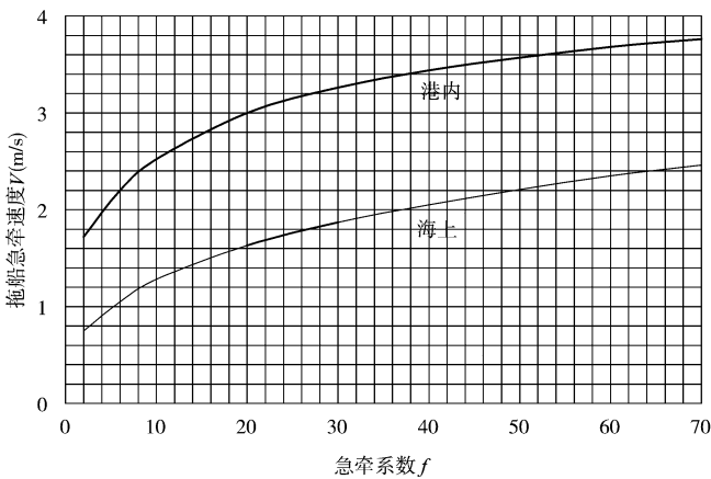
图 3.9.4 拖船急牵速度
