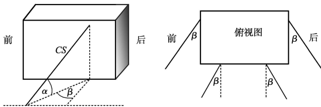
图 5(7) 垂向系固角 \alpha 和水平系固角 \beta
